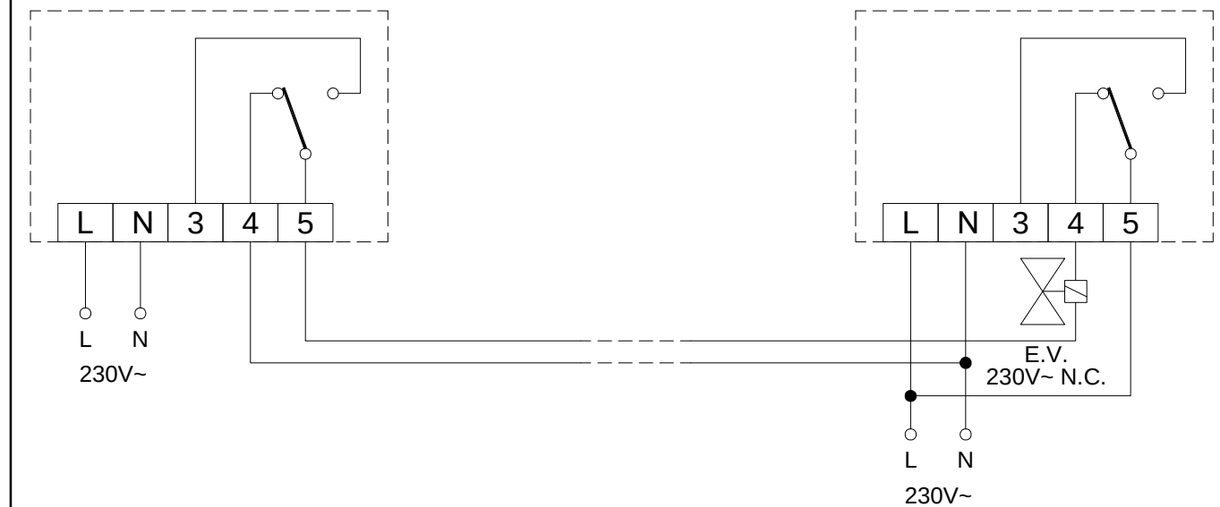
Fig. 4: Schema de legatura a mai multor Beagle cu o electrovana cu rearmare manuala, normal inchisa alimentare 230V~.
